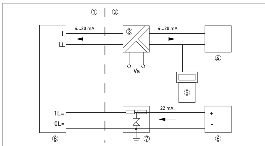
Рисунок 3-3: Пример подключения по 4-проводной схеме
