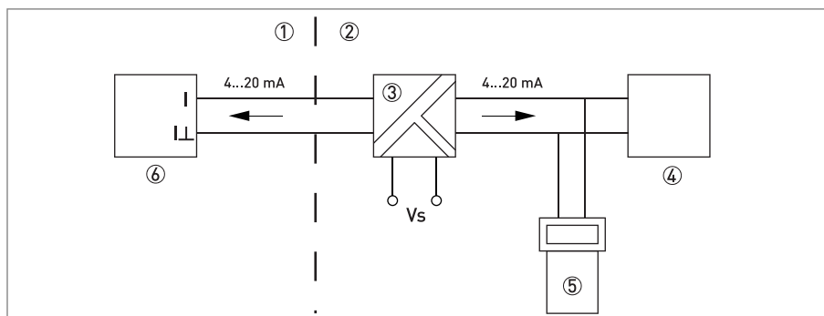
Рисунок 3-2: Пример подключения по 2-проводной схеме
