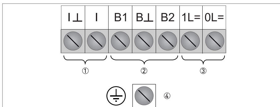
Рисунок 3-1: Клеммы OPTIFLUX 4040 C
