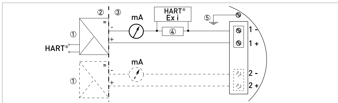
Figure 3-2: Schéma électrique pour équipement homologué Ex i avec option de sortie 4...20 mA
