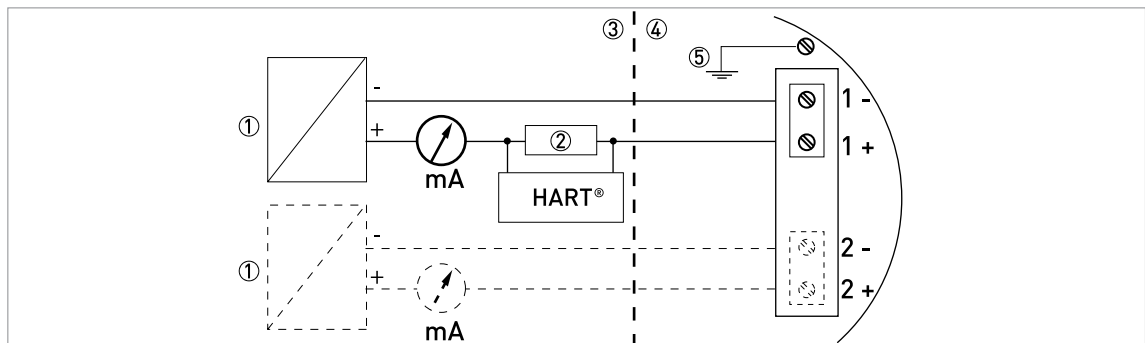
Figura 3-6: Esquema eléctrico para aparatos aprobados para Ex nA
