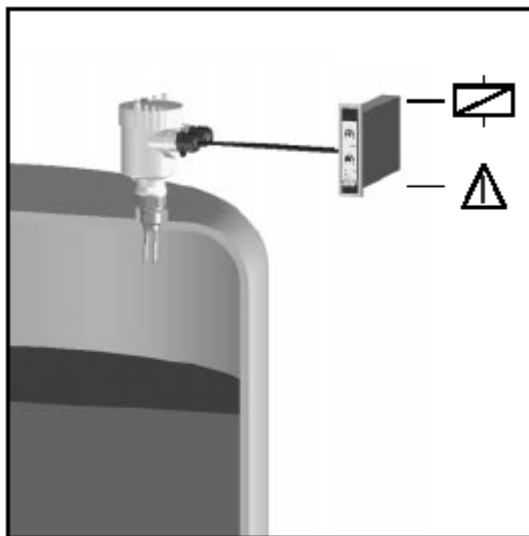
Měřicí systém s hladinovým spínačem s odděleným zpracováním
