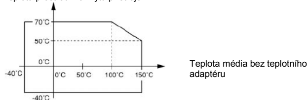
Teplota prostředí na krytu přístroje
