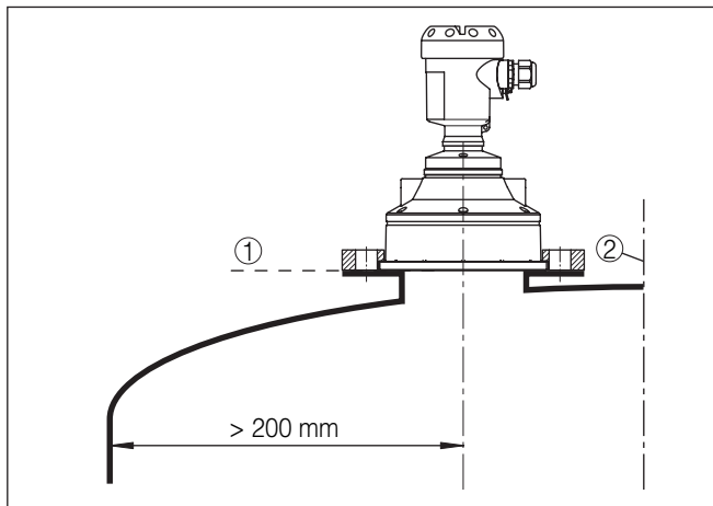
Abb. 5: Montage an runden Behälterdecken
