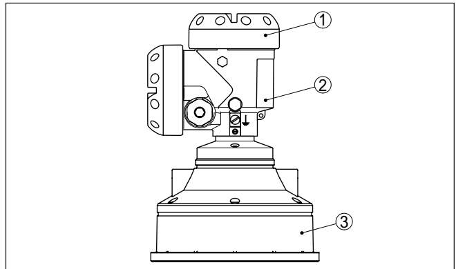
Abb. 1: OPTISOUND 3030 C, Aluminium-Zweikammergehäuse
