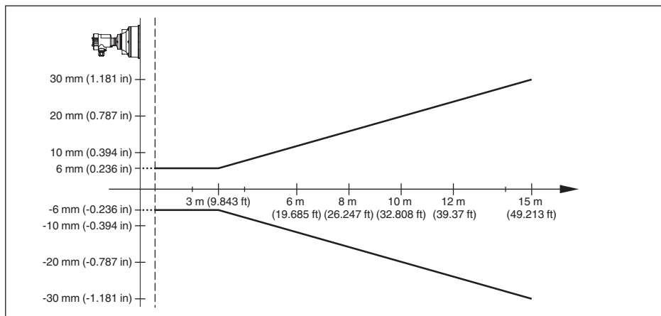
Abb. 24: Messabweichung OPTISOUND 3030 C
