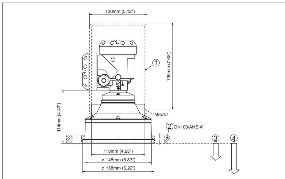
Abb. 26: OPTISOUND 3030 C
