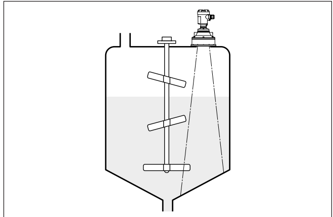
Abb. 12: Rührwerke
