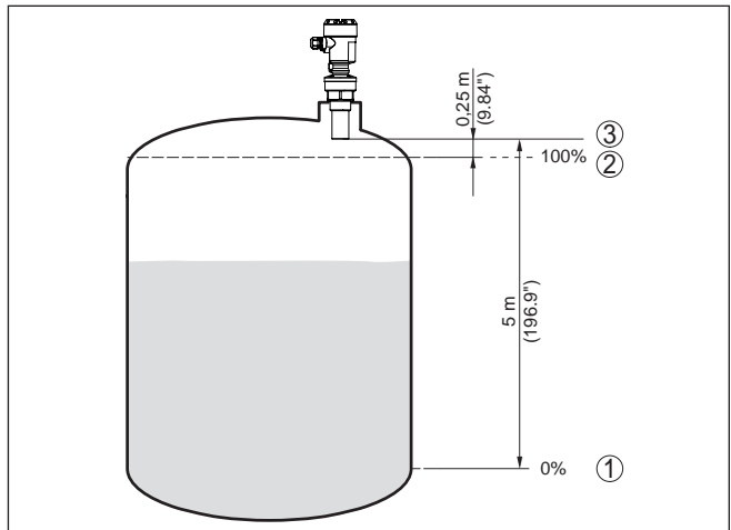
Abb. 22: Parametrierbeispiel Min.-/Max.-Abgleich
