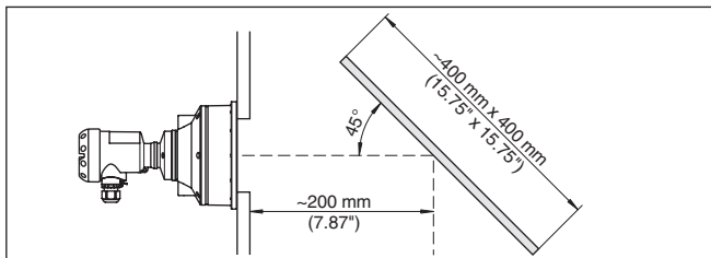
Abb. 10: Umlenkspiegel
