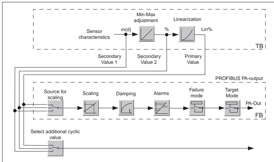
Fig. 26: OPTISOUND 3030 C: blokschema met AI (PA-OUT)-waarde en extra cyclische waarde
