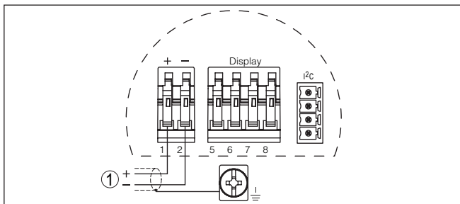
Fig. 17: Aansluitschema - eenkamerbehuizing
