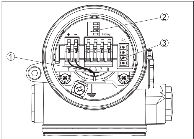
Fig. 19: Elektronicarimte tweekamerbehuizing
