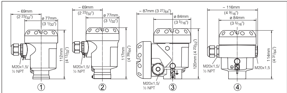
Fig. 29: Varianten behuizing in beschermingsklasse IP66/IP67 en IP66/IP68; 0,2 bar (met ingebouwde display- en bedieningsmodule wordt de behuizing 9 mm hoger resp. breder)
