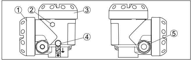
Fig. 18: Tweekamerbehuizing
