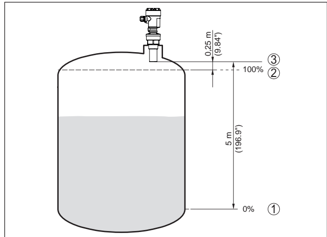
Fig. 24: Parametreervoorbeeld min./max.-inregeling
