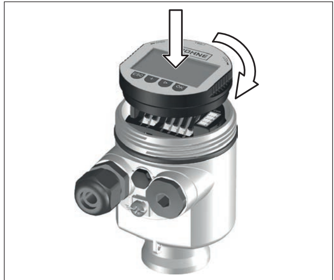
Fig. 22: Display- en bedieningsmodule in de eenkamerbehuizing plaatsen
