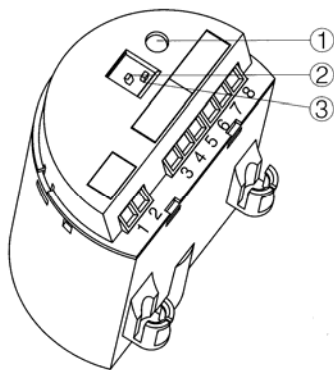
Obr. 10: Oscilátor SW E60R – reléový výstup
