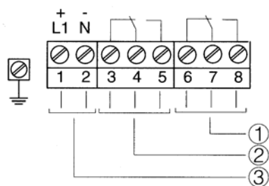
Obr. 9: Schéma zapojení, jednokomorové pouzdro
