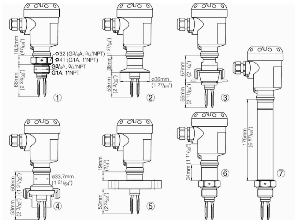
Obr. 15: Snimače OPTISWITCH 5100C, 5150C
