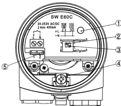
Obr. 9: Prostor elektroniky, jednokomorové pouzdro
