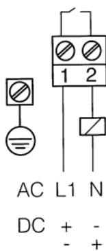
Obr. 9: Schéma zapojení, jednokomorové pouzdro
