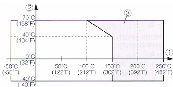
Obrázek č. 12: Diagram teplota prostředí – teplota měřeného média
