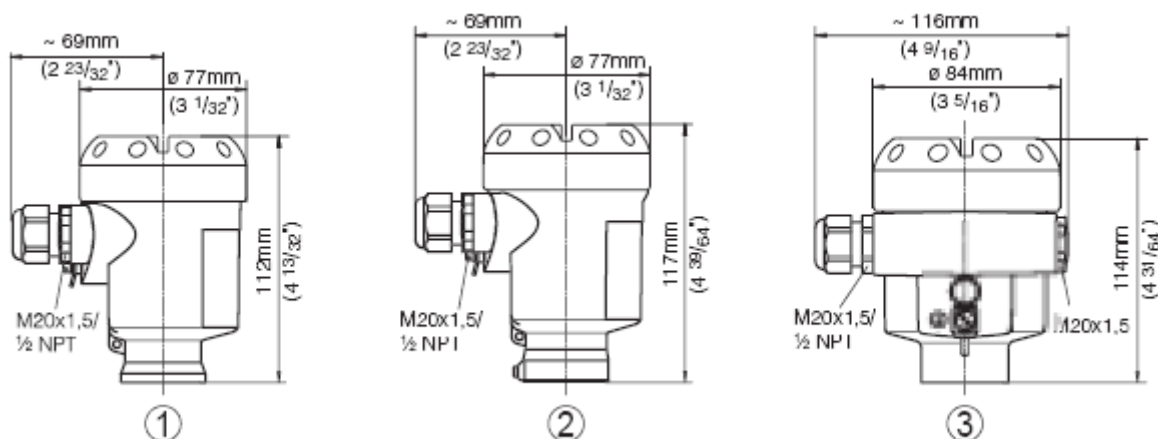
Rys. 13: Wersje obudowy
