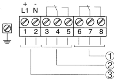
Obr. 11: Schéma zapojení, jednokomorové pouzdro
