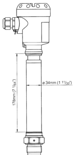
Obr. 16: Teplotní adaptér
