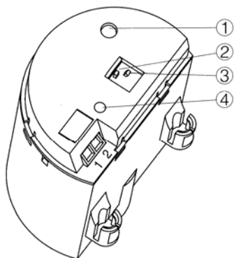
Obr. 12: Oscilátor SW E60N – výstup dle NAMUR
