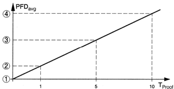
Obrázek č. 13: Závislost průběhu \text{PFD}_{\text{avg}} 1) na čase
