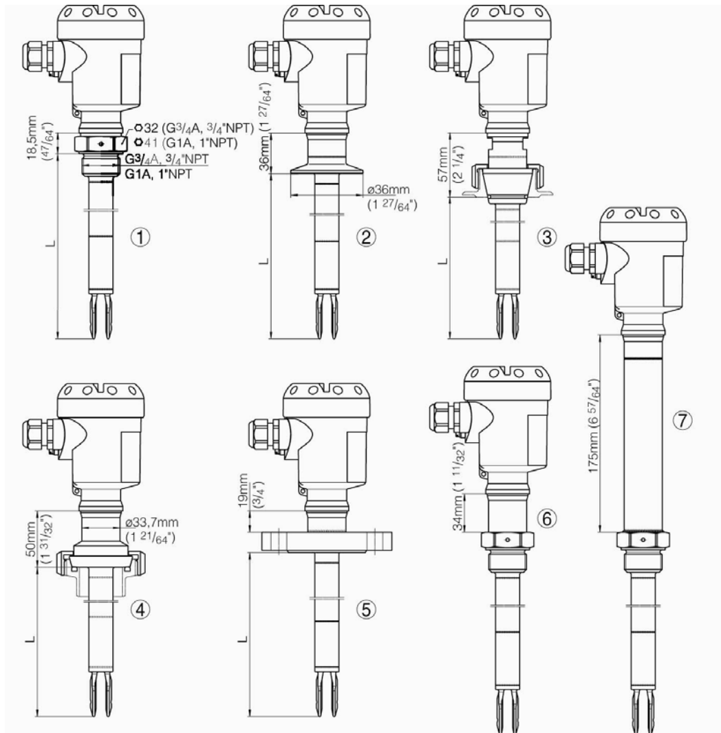
Obr. 17: Snímače OPTISWITCH 5200C, 5250C
