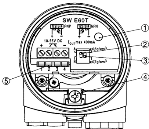
Obr. 10: Prostor elektroniky, jednokomorové pouzdro
