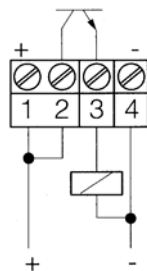
funkce PNP
