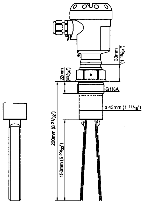
Obr. 19: OPTISWITCH 3100C se závitovým připojením G 1 1/2"
