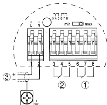
Obr. 11: Schéma zapojení
