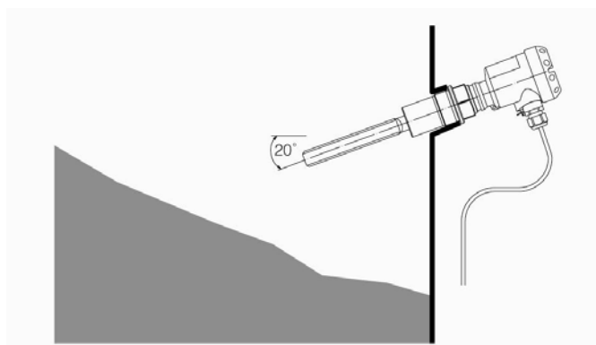
Obr. 4: Vodorovná montáž
