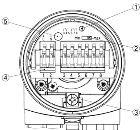
Obr. 10: Prostor elektroniky
