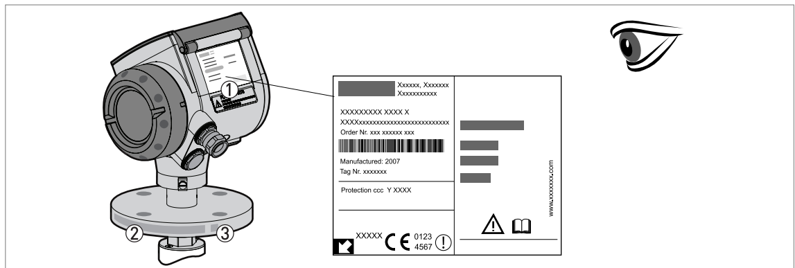
Kuva 2-3: Silmämääräinen tarkastus
